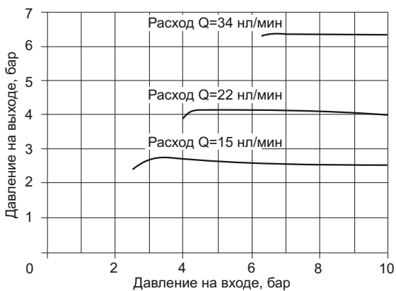
Регулировочные характеристики
